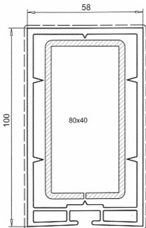
Vorsatzzarge 58x100mm
