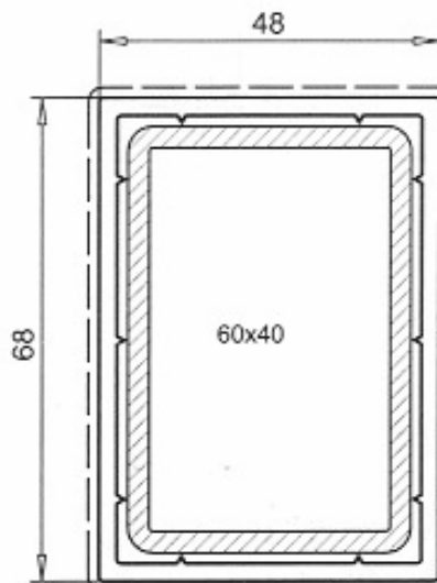
Vorsatzzarge 48x68mm
