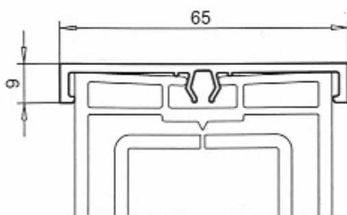
Abdeckprofil
