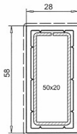
Vorsatzzarge 28x58mm
